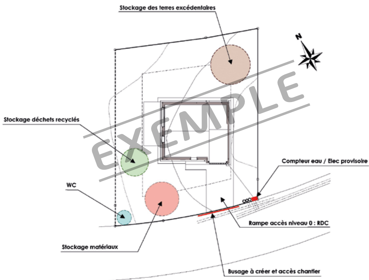
Exemple de PIC réalisé à partir du plan de masse
